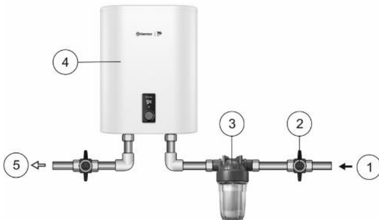
Рис.2 Схема подключения фильтра.
