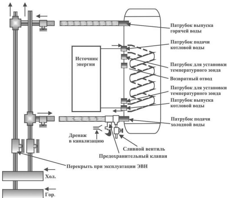
Рисунок 1. Схема подключения.
