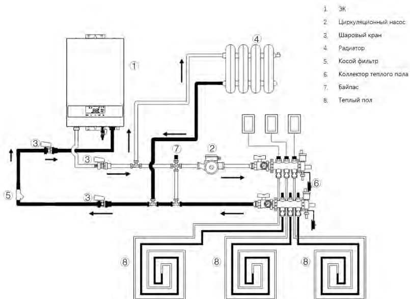
Рис. 14. Схема подключения «ЭК + Теплый пол».
