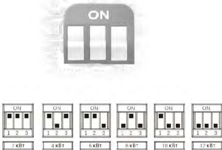
Рис. 8. Положение рычагов переключателя мощности.
