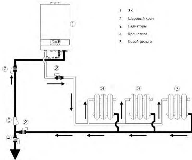
Рис. 13. Схема подключения «ЭК + Радиаторы».
