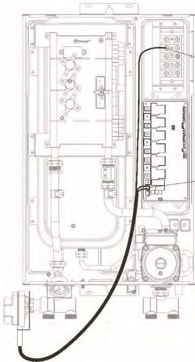
Рис. 17. Подключение трехходового клапана
