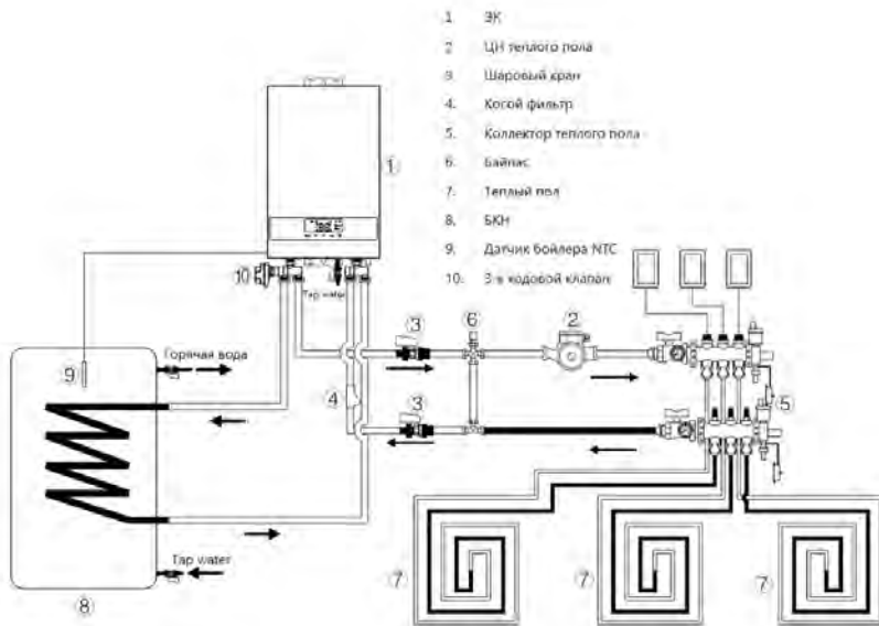
Рис. 20. Схема подключения «ЭЖ + БКН + Теплый пол».
