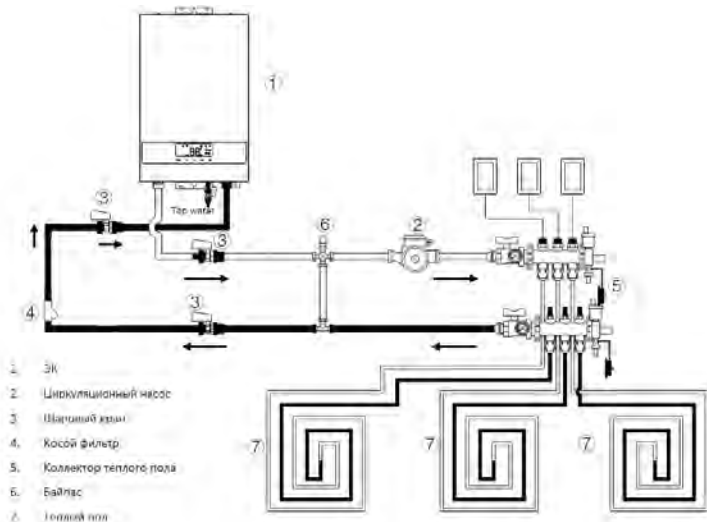
Рис. 14. Схема подключения «ЭК + Теплый пол».
