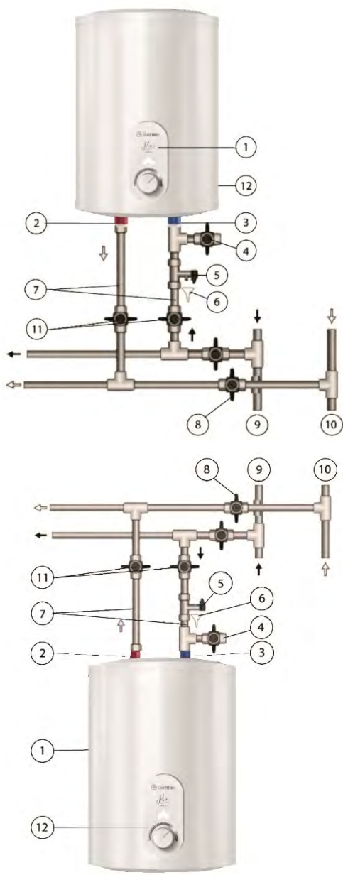
Рисунок 1. Схема подключения
