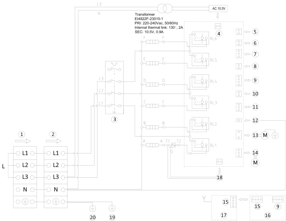
Рис. 13. Электрическая схема подключения контактов к плате управления PCB
