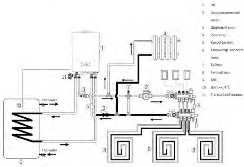
Рис. 16 Схема подключения «ЭЖ + БКН + теплый пол»
