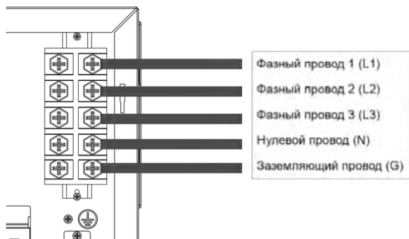
Рис. 11. Трехфазное подключение прибора
