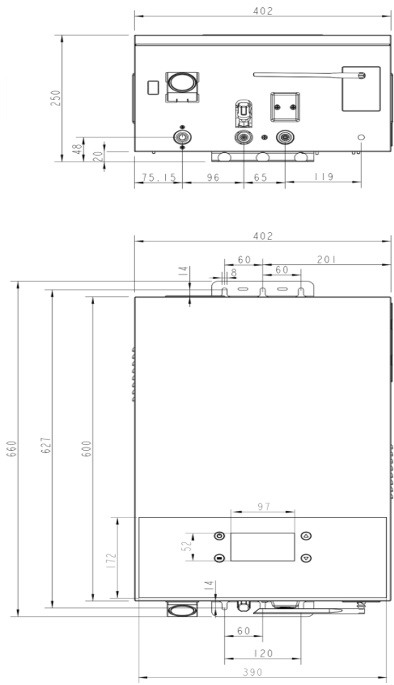
Рис.2. Габаритные размеры
