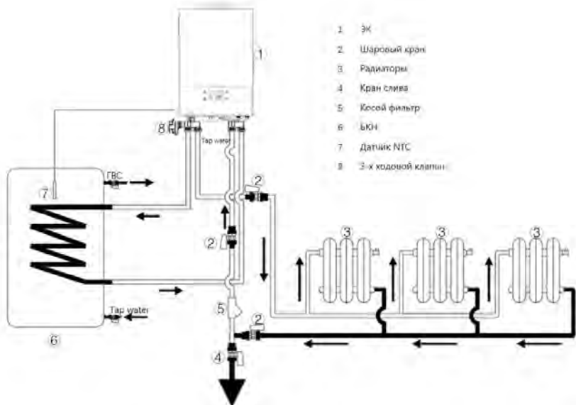
Рис. 15 Схема подключения «ЭК + БКН + радиаторы»
