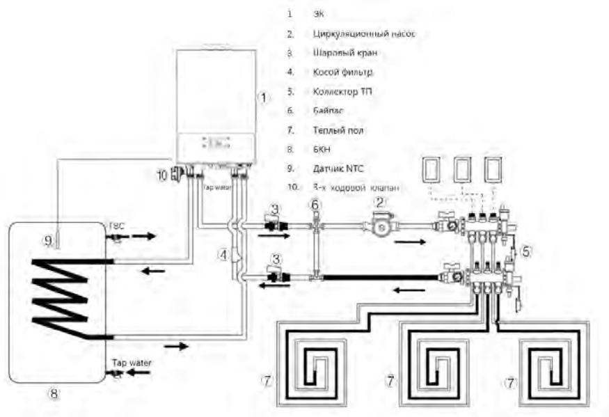
Рис. 16 Схема подключения «ЭЖ + БКН + теплый пол»
