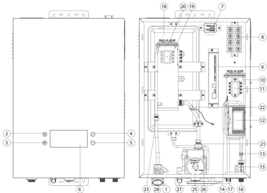
Рис. 1. Конструкция изделия
