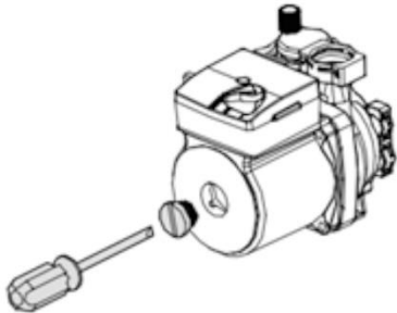
Рис. 16. Проверка насоса
